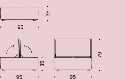
TRAY ELEMENT ABLAGEELEMENT
